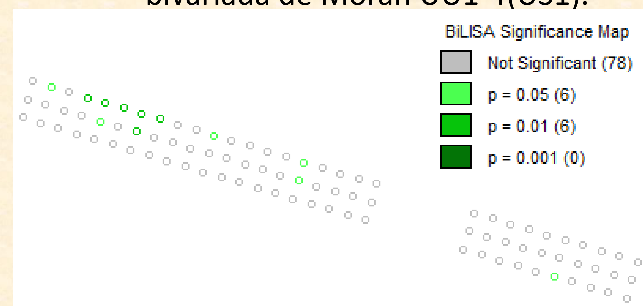
Figura 4: Mapa de significância dos índices de bivariada de Moran UU1=f(US1).
