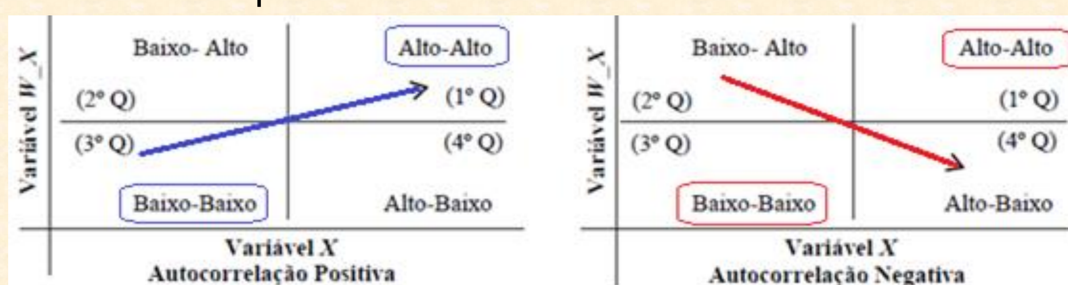
Figura 1: Diagrama de dispersão de Moran.
