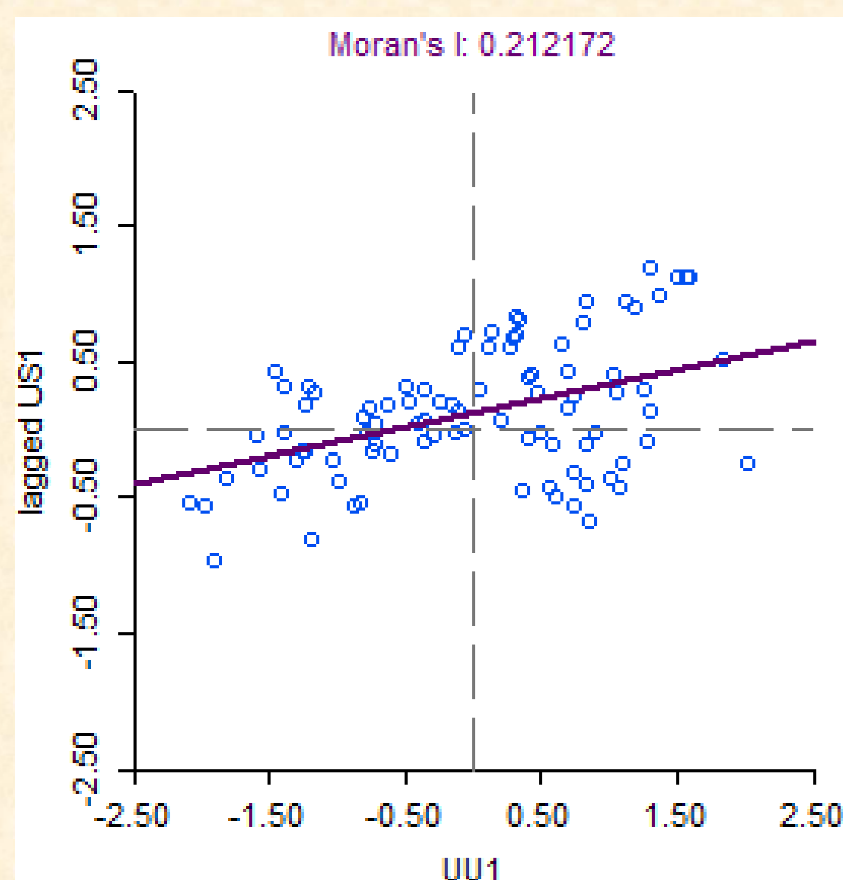
Figura 2: Diagrama de Dispersão de Moran entre UU1=f(US1).
