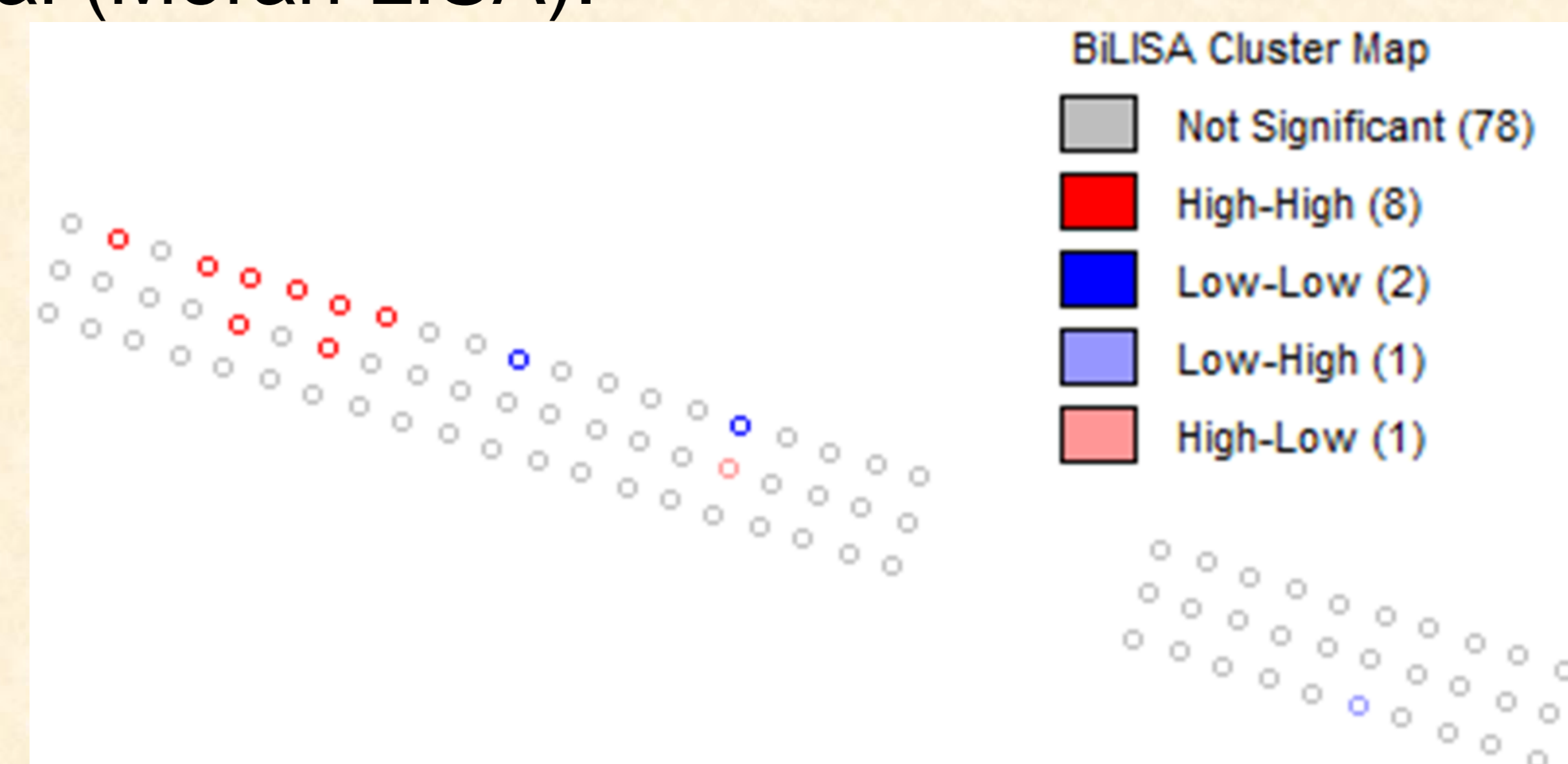
Figura 3: Mapa de cluster dos índices de bivariada de Moran UU1=f(US1).
